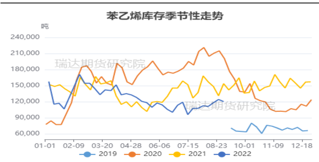
图15、苯乙烯库存
