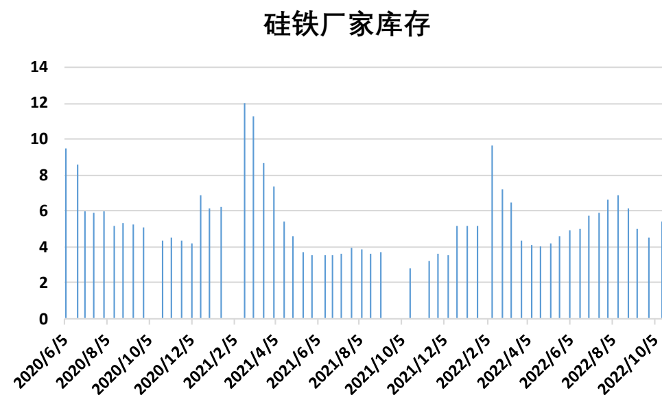
图10、硅铁库存
