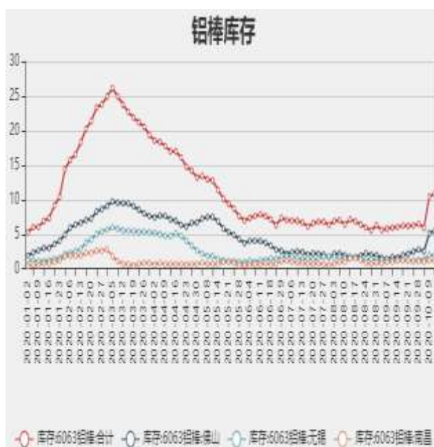
图6：铝棒库存
