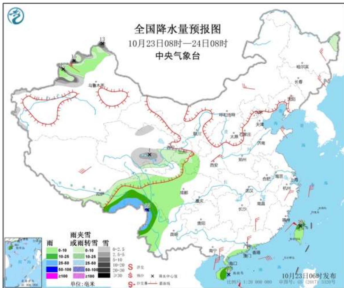
图：全国降水量预报图
