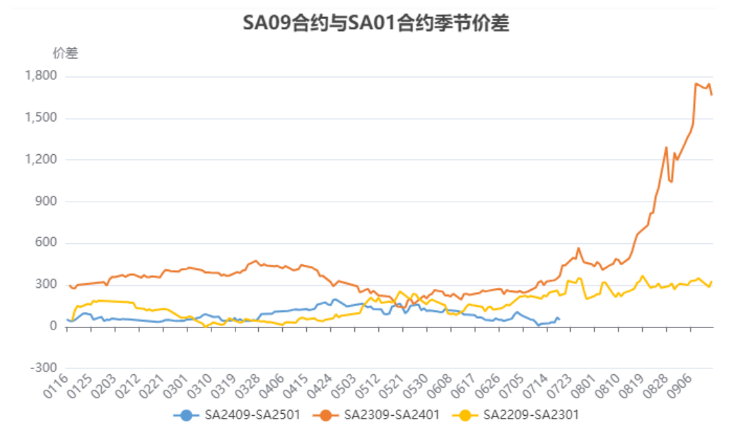
SA 9-1价差
