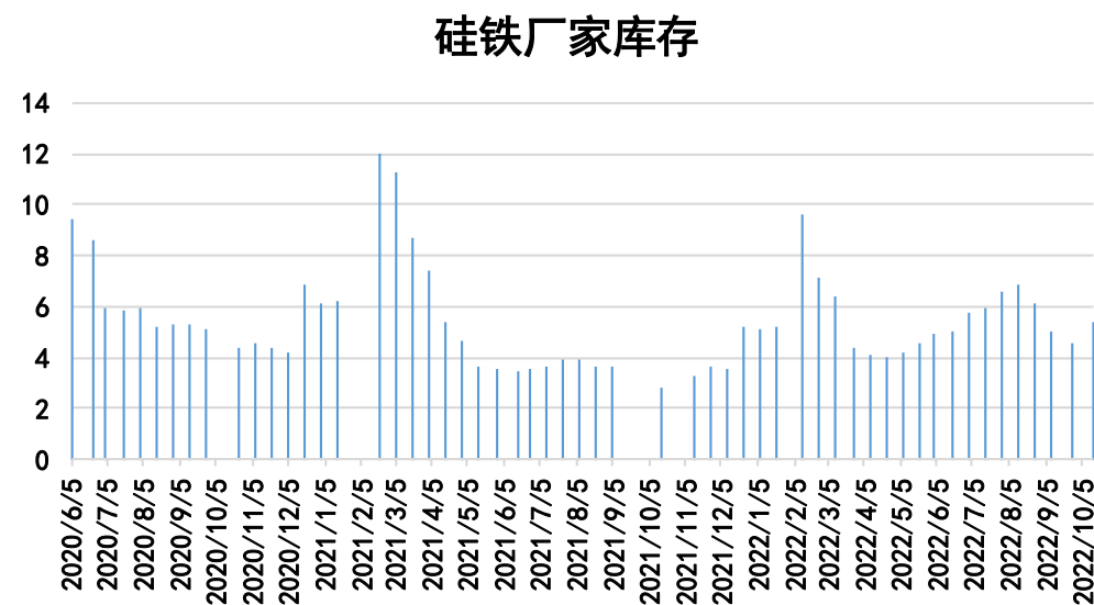
图10、硅铁库存
