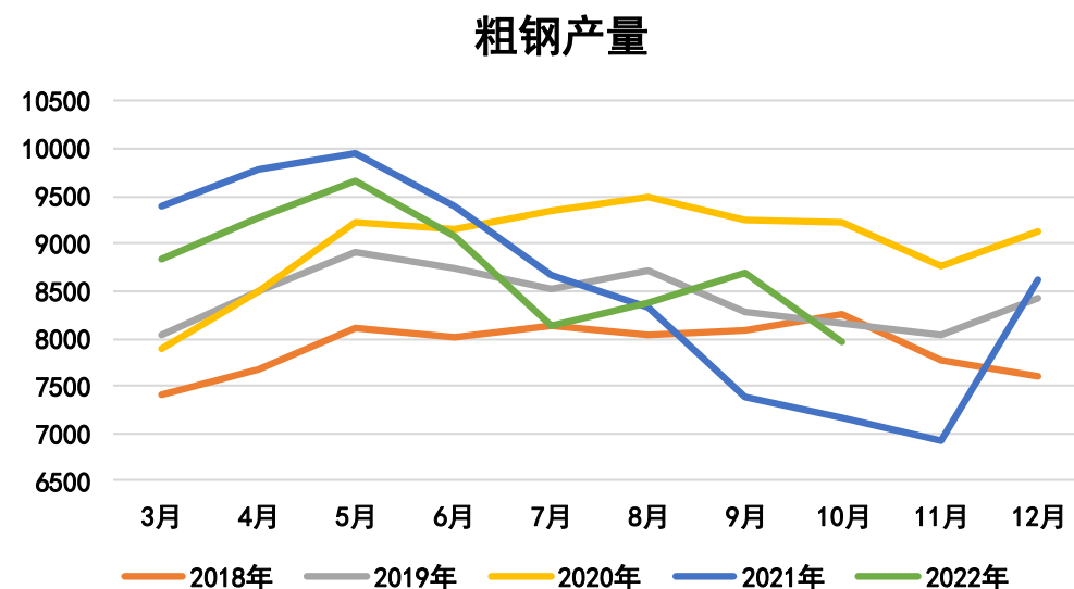
图15、粗钢产量
