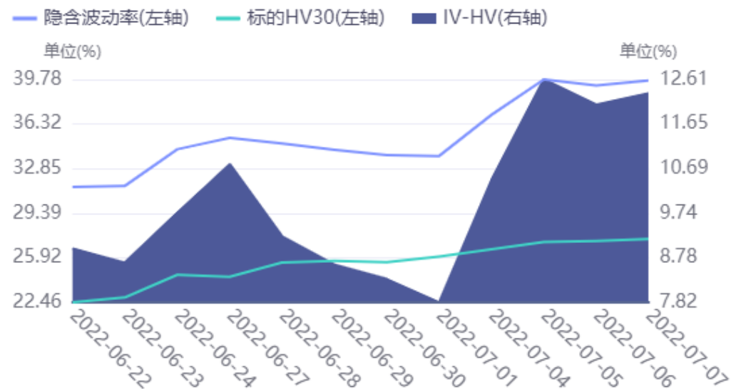
图24、隐含波动率
