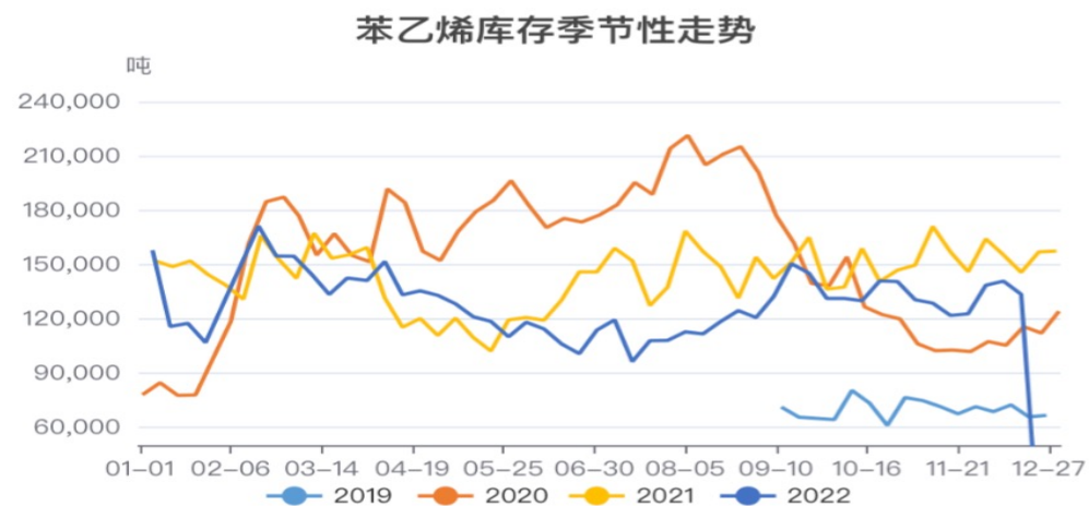
图15、苯乙烯库存
