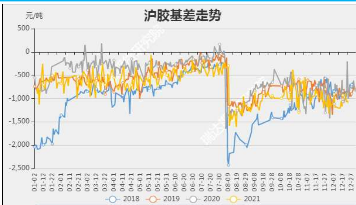
图4 沪胶基差
