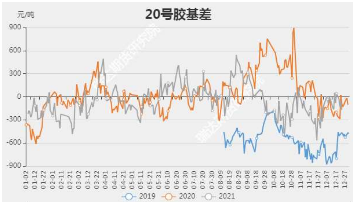
图5 20号胶基差
