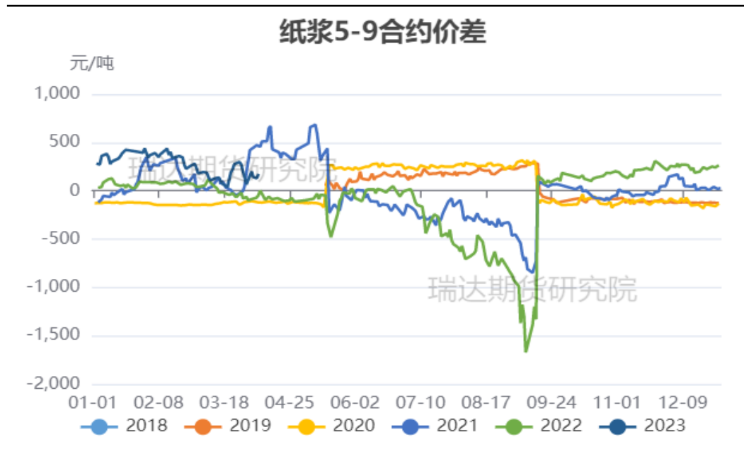
图、纸浆近远月走势图
