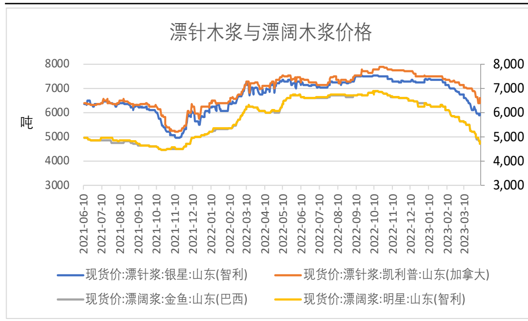
图、漂针木浆与漂阔木浆价格
