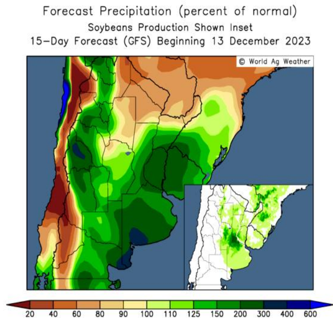
图 阿根廷未来15天降水距平 (%)
