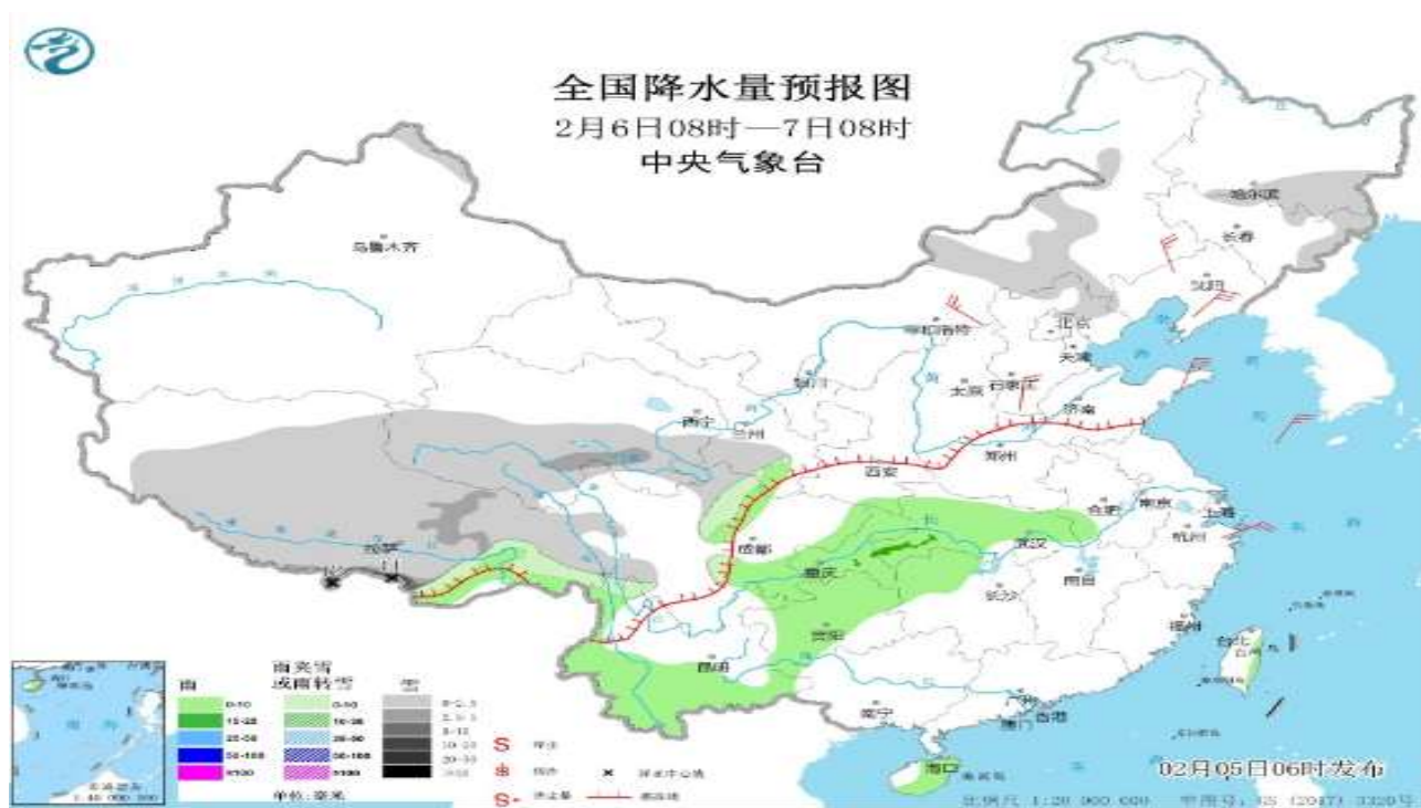
图：全国降水量预报图
