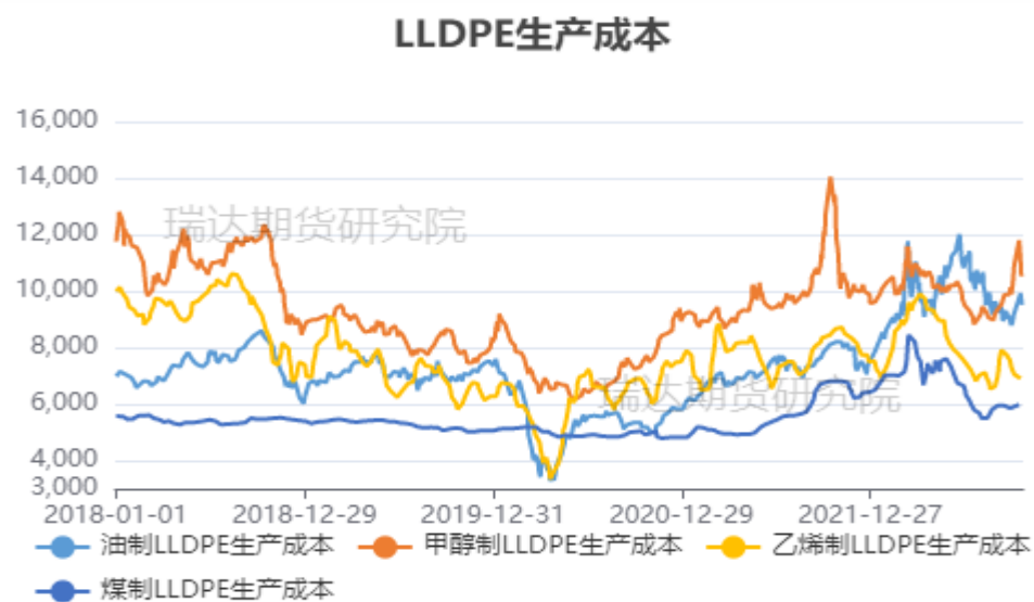
图15、聚乙烯生产成本
