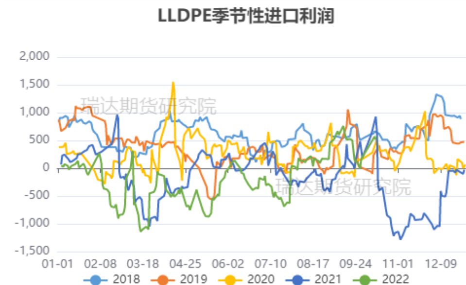
图19、聚乙烯进口成本利润
